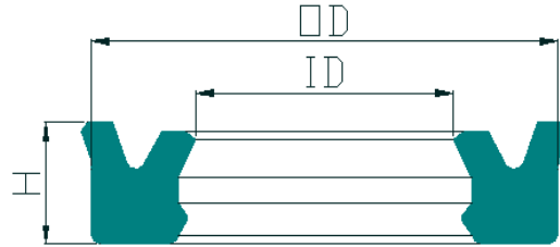
TYPE - HP4
